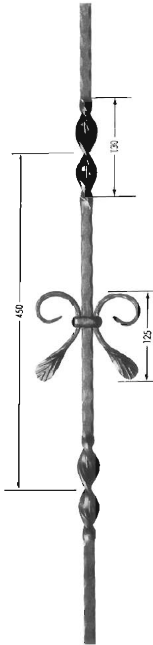
4-5213 L: 950 mm. Ø 14 mm.
