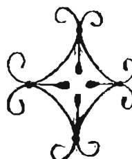
4-2782 Medidas: 425 x 425 mm. Material: 12 x 6 mm.
