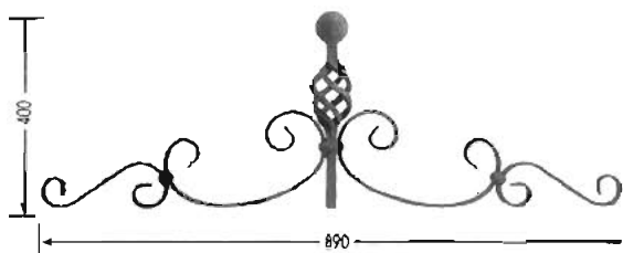
4-2302 Medidas: 890 x 400 mm. M: 12 x 6 mm.
