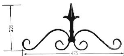
4-2309 Medidas: 475 x 235 mm. M: 12 x 6 mm.
