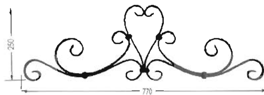
4-2308 Medidas: 770 x 250 mm. M: 12 x 6 mm.
